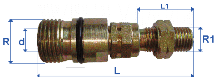
CUERPO ACOPLE LENTO ROSCA INTERIOR CIERRE VALVULA EN PUNTA
