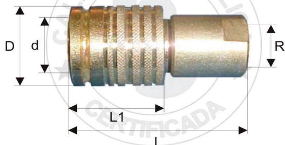
CUERPO ROSCA INTERIOR - ESPECIAL VALMET
