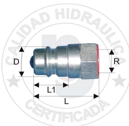
NIPLE ROSCA METRICA INTERIOR ASIENTO ARANDELA
