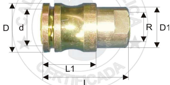
CUERPO ROSCA INTERIOR ASIENTO AROSELLO (O' ring)
