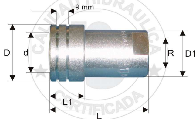
CUERPO ROSCA CONICA INT. AS.AROSELLO (O'ring)- ESPECIAL ZANELLO MOD.NUEVO
