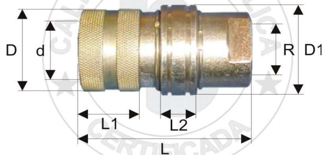
CUERPO ROSCA CONICA INTERIOR 1/2 NPT
