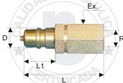
NIPLE ACOPLE ESPECIAL PLATAFORMA COSECHADORA - ROSCA METR. INT.
