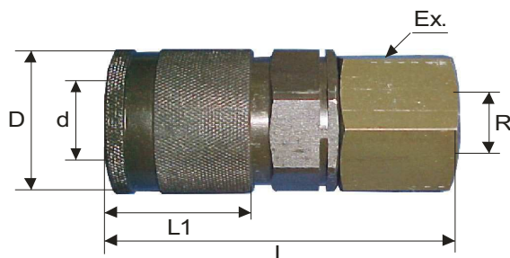
CUERPO ROSCA INTERIOR METRICA
