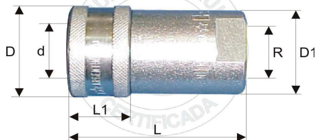
CUERPO ROSCA CONICA INTERIOR
