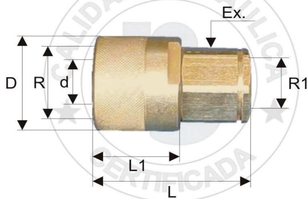
NIPLE ACOPLE CIERRE VALVULA EN PUNTA - ADAPTACION BOBCAT
