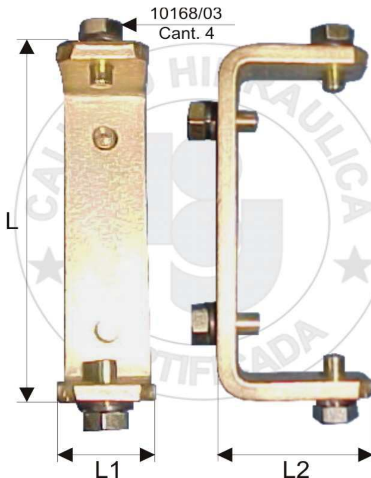
FIJACION "U" PARA SOPORTE DOBLE
