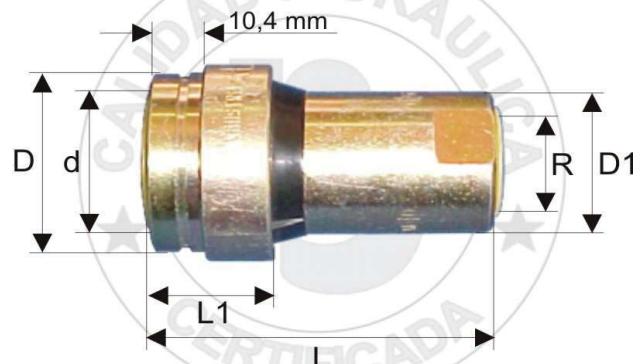
CUERPO ROSCA INTERIOR ASIENTO AROSELLO (O'ring) - ESPECIAL FIAT IMP.MOD.VIEJO
