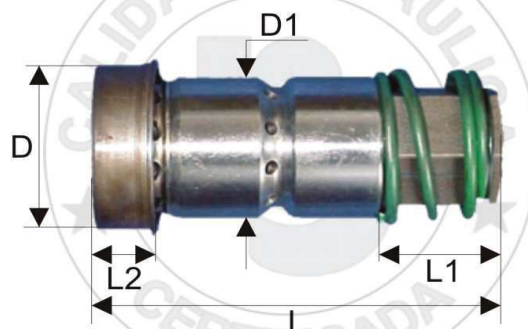
CUERPO ACOPLE HIDRAULICO INTEGRAL JOHN DEERE
