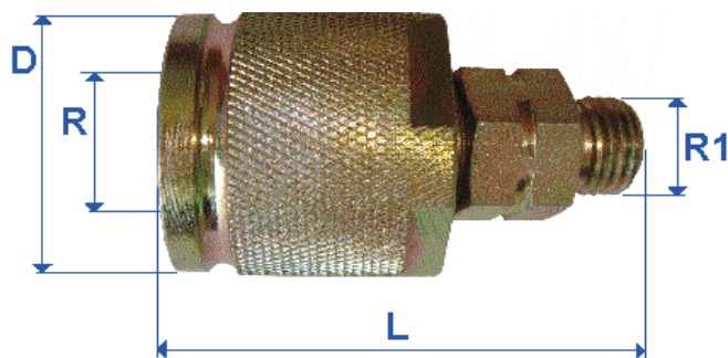
NIPLE ACOPLE LENTO ROSCA INTERIOR CIERRE VALVULA EN PUNTA
